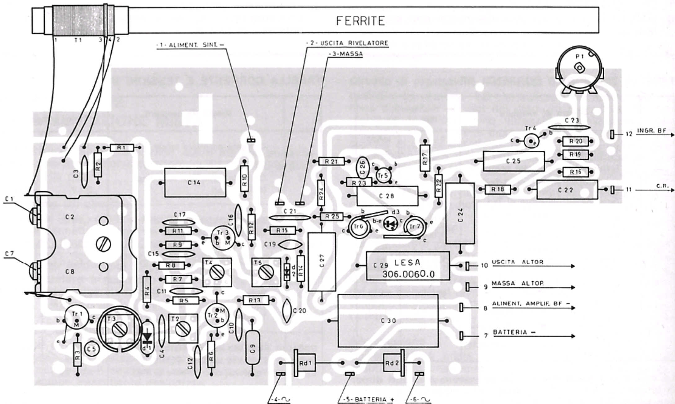
Circuito stampato Mod. 416/R.
